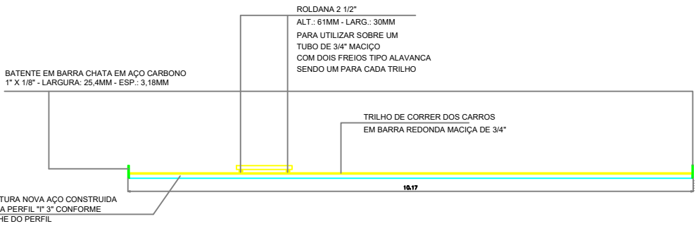
DETALHE - CARR0 DE MOVIMENTAÇÃO VISTA LATERAL
