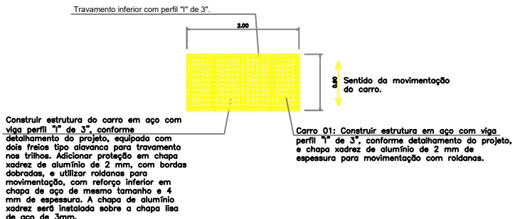
DETALHE - CARR0 DE MOVIMENTAÇÃO VISTA SUPERIOR
