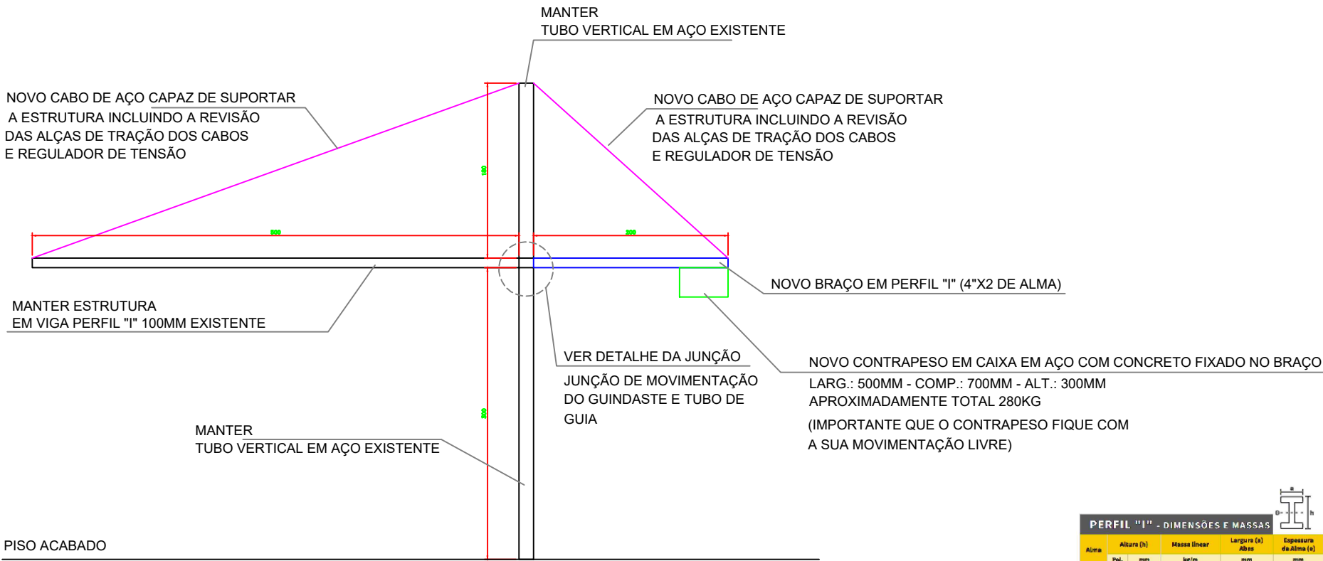
DETALHE - GUINDASTE DE MANUTENÇÃO DA CAG
