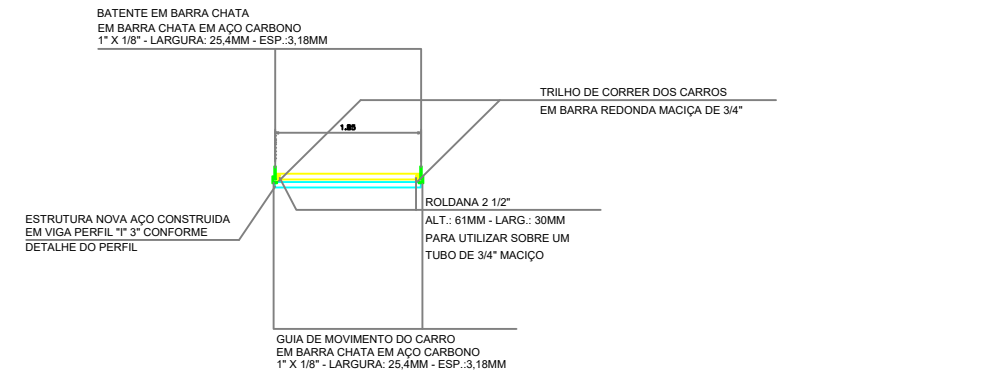
DETALHE - CARR0 DE MOVIMENTAÇÃO VISTA FRONTAL
